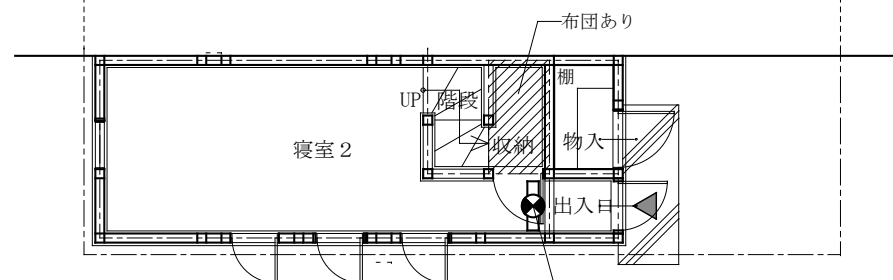
地階平面図 S:1/100
